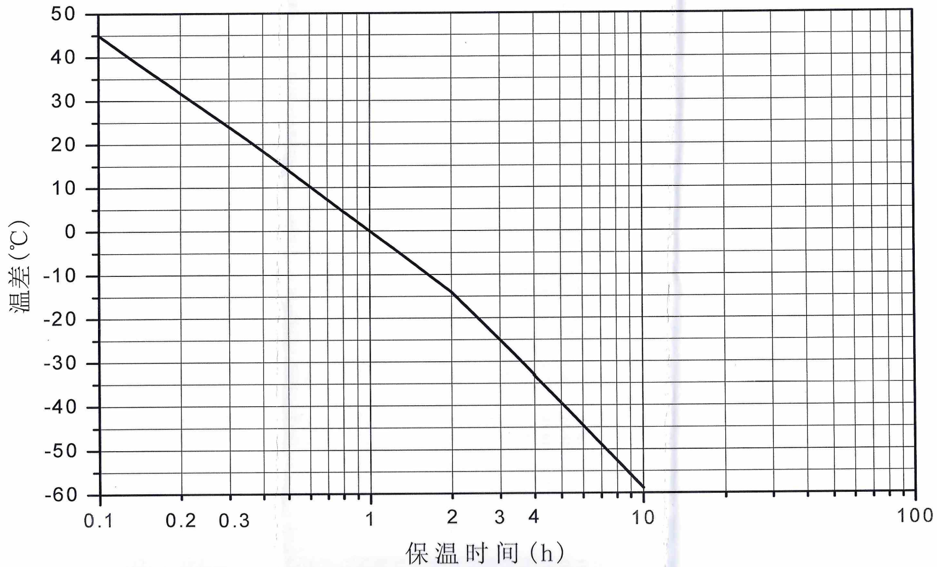
BTC温度校正曲线 (900°C - 1200°C)
