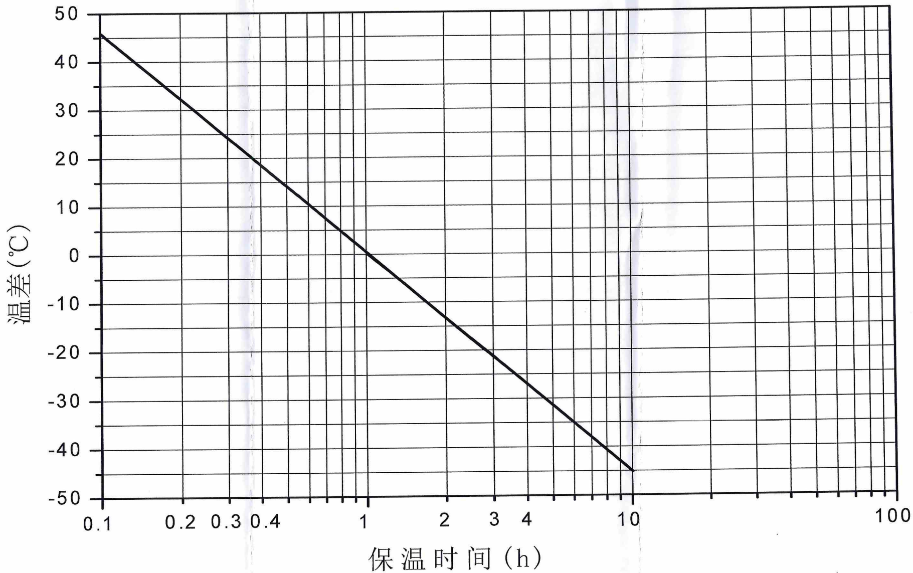
CTC温度校正曲线 (1100℃ - 1400℃)
